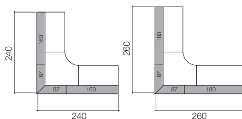
Eckkombination mit Verkettungsplatte
