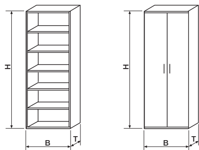
Breiten-, Höhen- oder Tiefenkürzung bei Anbauteilen
